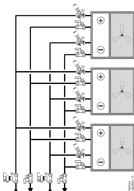
Fan coils
